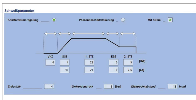
▲ Programmierung – Eingabe der Schweißparameter
